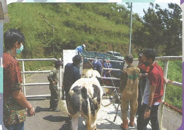
Distribusi Calon Pejantan Unggul ke BIB Lembang
